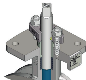
Lange Stopfbuchse zur Positionierung
