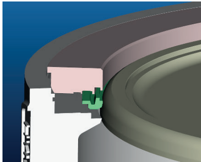
Modifizierter PTFE-Sitz
