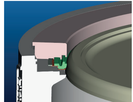
Feuerfester Sitz
