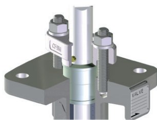
Stopfbuchsenflansch und Stopfbuchse
